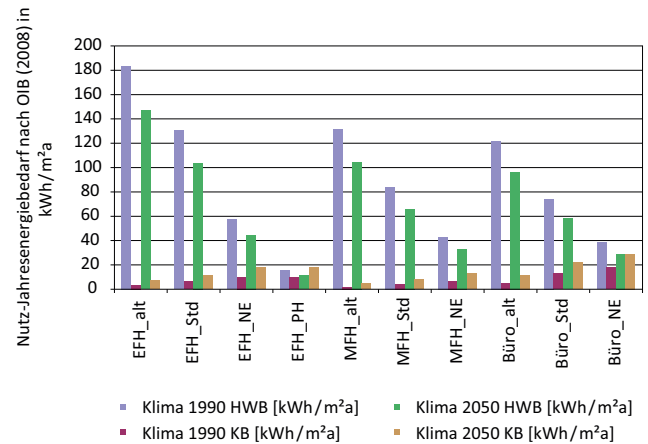
Abbildung 5.23 Spezifischer Heizwärmebedarf (HWB) und Kühlbedarf (KB) für Referenzgebäude am Beispiel des Klimas Graz in kWh/m²/Jahr; EFH: Einfamilienhaus, MFH: Mehrfamilienhaus, PH: Passivhaus, Büro: Bürogebäude. Quelle: Gobiet et al. (2009)
