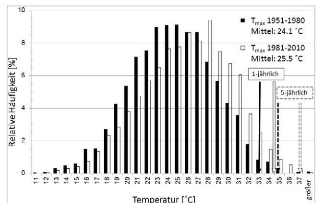
Abbildung 5.6 Häufigkeitsverteilung der Maximalen Sommertemperaturen an der Station Wien, Hohe Warte, in den Monaten Juni, Juli und August für die Zeiträume 1951 bis 1980 und 1981 bis 2010. Datenquelle: ZAMG
