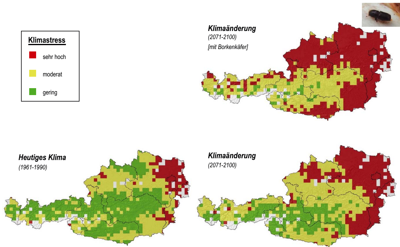
Abbildung 3.4 Modellerter Klimastress für die Fichte basierend auf dem Konzept der physiologischen Nische. Datenbasis: Standortdaten der Österreichischen Waldinventur (ohne Schutzwald außer Ertrag). Links unten: Heutiges Klima repräsentiert durch die Messperiode 1961 bis 1990; rechts unten: Klimaänderungsszenario A1B am Ende des 21. Jahrhunderts (Temperatur: bis +4,5°C, Niederschlag: bis –35 % im Sommerhalbjahr); rechts oben: Klimaänderungsszenario A1B, physiologische Nische plus Berücksichtigung der potentiellen Generationen des Fichtenborkenkäfers Ips typographus . Rot = Klimastress sehr hoch, gelb = Klimastress moderat, grün = Klimastress gering bzw. nicht vorhanden
