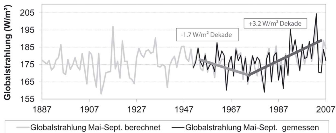
Abbildung 5.7 Zeitlicher Verlauf der Globalstrahlung für die Periode Mai-September an der Station Wien, Hohe Warte, aus Messungen seit 1951 und mittels empirischer Formel berechnet aus der Sonnenscheindauer. Datenquelle: ZAMG
