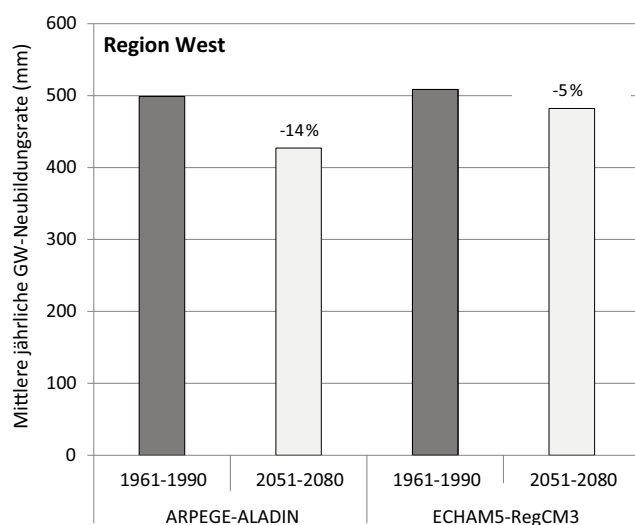
Abbildung 2.28 Änderung der mittleren jährlichen Grundwasserneubildungsrate der Periode 2051–2080 bezogen auf den Referenzzeitraum 1961–1990 für die Auswerteregionen West, Ost und Süd. Quelle: Nachtnebel et al. (2012)
