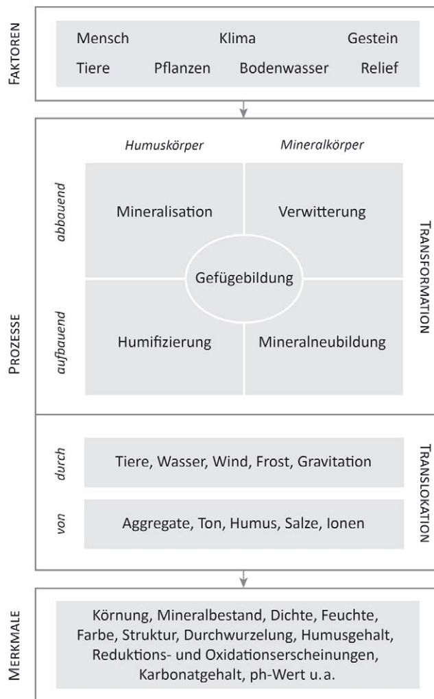
Abbildung 5.1 Schematischer Überblick zu den bodenbildenden Faktoren und Prozessen und den sich daraus ergebenden Merkmalen des Bodens. Die Vielfalt an Faktoren und Prozessen sowie ihrer Kombinationsmöglichkeiten lassen erahnen, wie schwer die Zusammenhänge im System Boden zu identifizieren und zu quantifizieren sind. Erstellt von Geitner für AAR14
