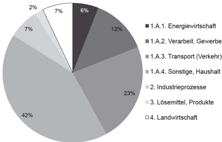
Abbildung 2.5 Aufteilung der PM2.5 Emissionen Österreichs (2010) nach 'NFR' Quellgruppen Figure 2.5 Partitioning of PM2.5 emissions in Austria (2010) according to 'NFR' source sectors
