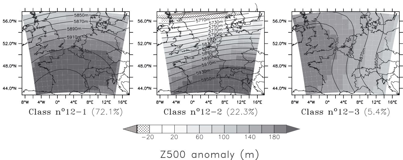
Abbildung 4.2 Anomalien der geopotentiellen Höhe auf dem Druckniveau 500 hPa im Globalmodell HadGEM1 bei Verwendung des Szenarios SRES A1B (2081–2100 minus 1961–1990). Über Westeuropa kommt es zu einem Druckanstieg durch das sich nach Osten ausdehnende Azorenhoch. Adaptiert nach Belleflamme et al. (2011)
