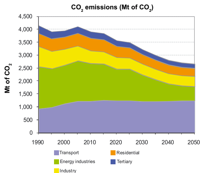
Abbildung 3.31 Entwicklung der direkten CO 2 -Emissionen aller Sektoren bis 2050 (EU27) (Quelle: European Commission, EC (2011b))
